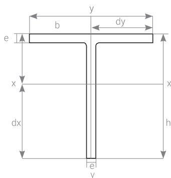
Perfil T
