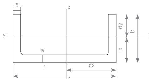
Perfil U
